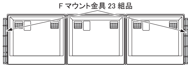
3台連結（背面）
